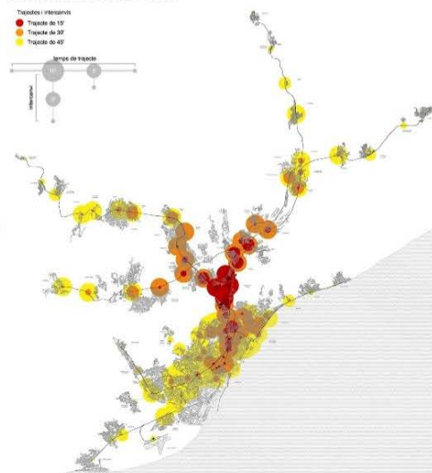
ACCESSIBILITAT FERROVIÀRIA
